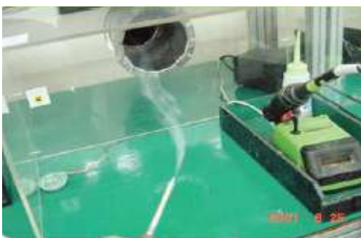
발연관을 이용한 기류 확인
